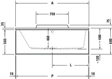
# 700292 00 0 00 0000, 1600 x 700 mm # 700294 00 0 00 0000, 1700 x 700 mm # 700296 00 0 00 0000, 1700 x 750 mm Mit optionaler Wannerverkleidung.* With optional bathtub panel.* Con pannello optional*
