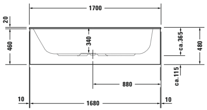
# 700231 00 0 00 0000, 1700 x 750 mm Mit optionaler Wannerverkleidung.* With optional bathtub panel.* Con pannello optional*
