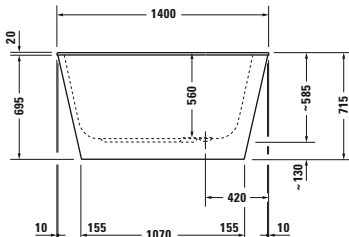
# 700233 00 0 00 0000, 1400 x 800 mm Mit optionaler Wannerverkleidung.* With optional bathtub panel.* Con pannello optional*
