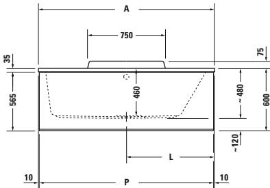
# 700293 00 0 00 0000, 1600 x 700 mm # 700295 00 0 00 0000, 1700 x 700 mm # 700297 00 0 00 0000, 1700 x 750 mm Mit optionaler Wannerverkleidung.* With optional bathtub panel.* Con pannello optional*
