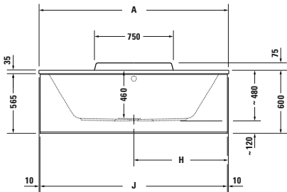
# 700298 00 0 00 0000, 1800 x 800 mm # 700299 00 0 00 0000, 1900 x 900 mm Mit optionaler Wannerverkleidung.* With optional Bathtub panel.* Con pannello optional*
